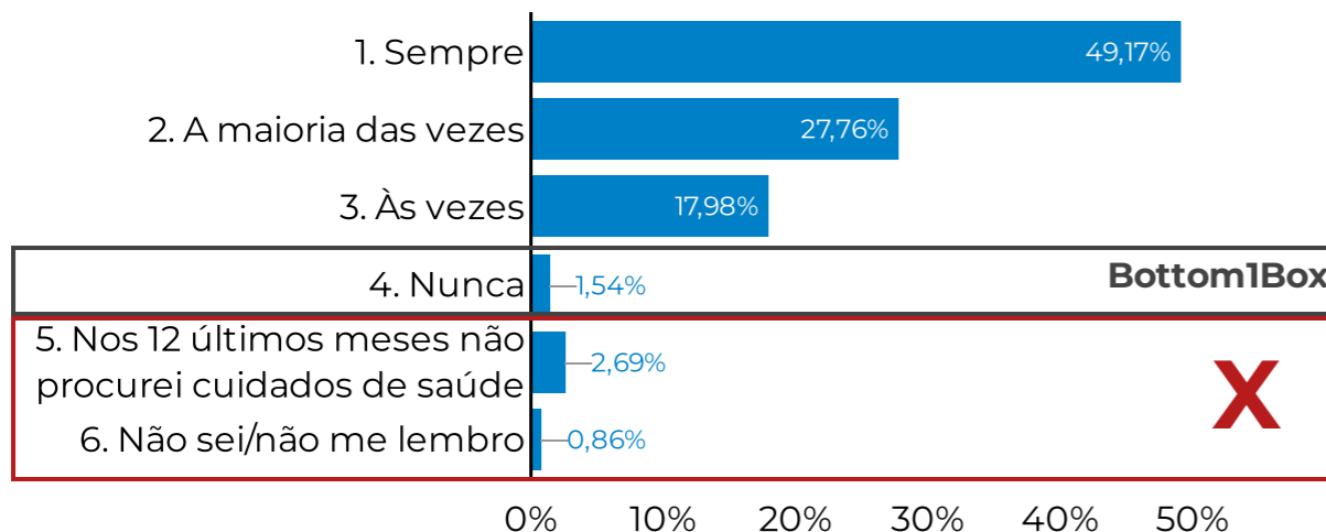
Gráfico 1 - Bottom1Box
